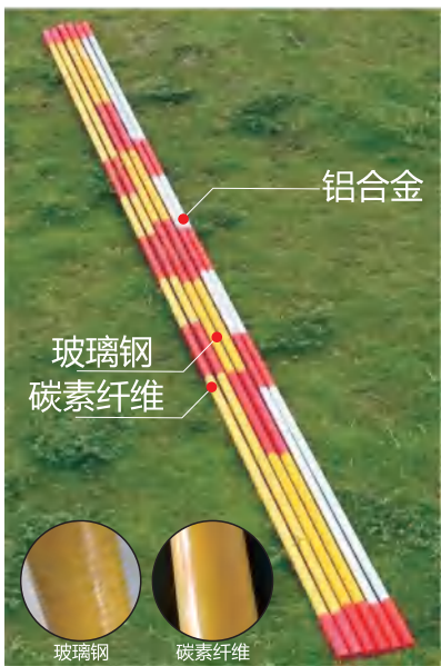
SC-88037 跳高横杆-铝合金 /玻璃钢/碳素纤维 High jump bar-Aluminum /FRP/Carbon fiber Product size: 4m (length) *3cm (diameter) 建议零售价：¥225/250/550/pc
